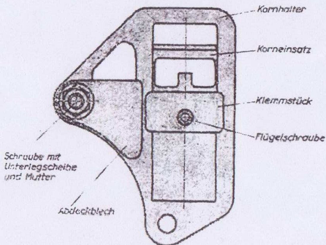
Verstellbares Korn mit Abdeckblech im Kornhalter eingebaut.
